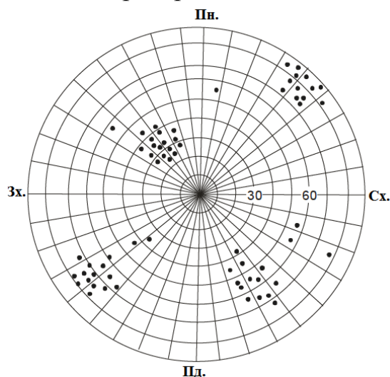
Рис. 2. - Точкова діаграма тріщинуватості
