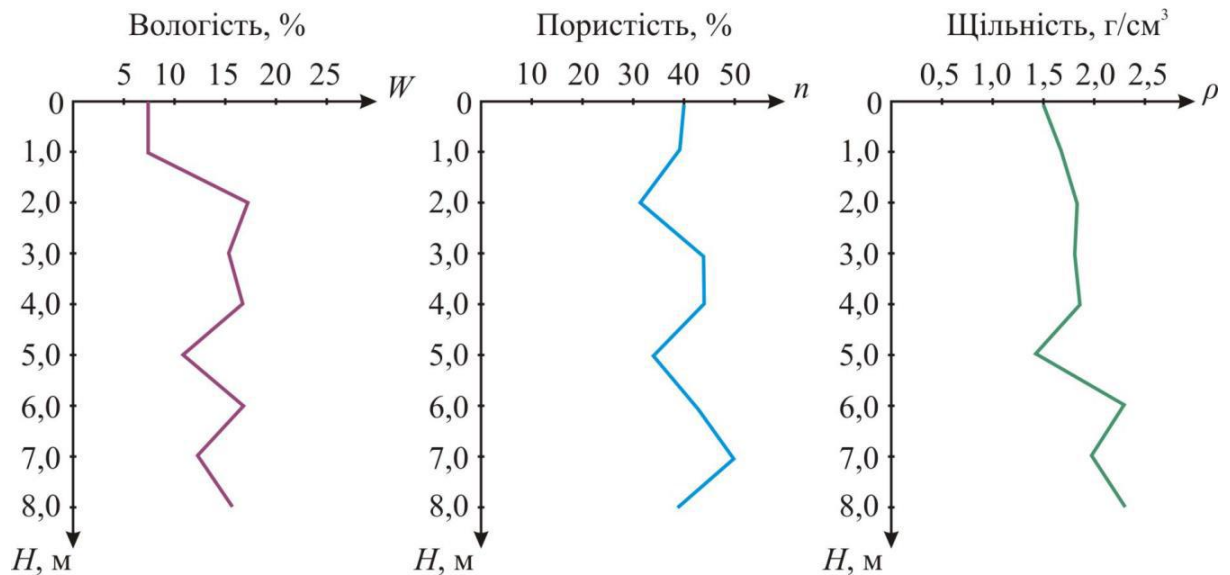
Рис. 1. Графік зміни фізичних властивостей ґрунту по глибині
