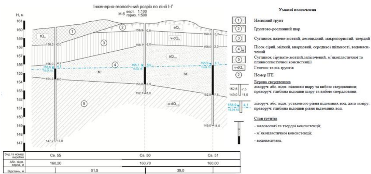
Рис. 1. Приклад інженерно-геологічного розрізу
