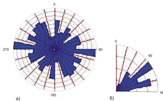
Рис. 1. Роза-діаграма тріщинуватості
