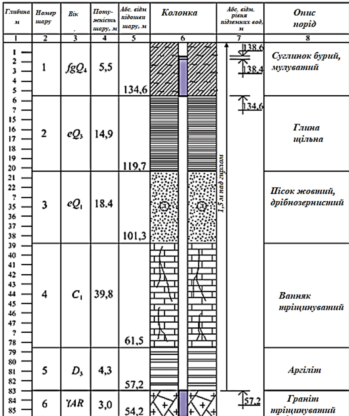
Рис. 1. Геологічна колонка бурової свердловини
