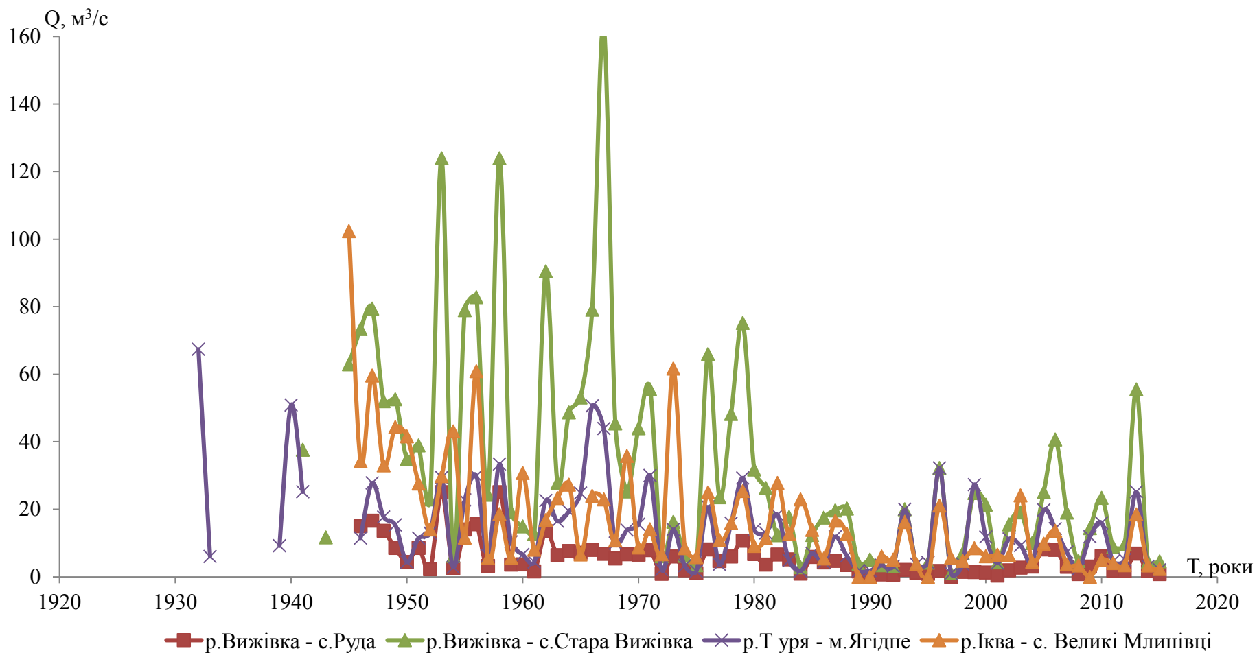
Рисунок Т.1 – Хронологічний графік ходу максимальних витрат води весняного водопілля в басейні р. Прип'ять
